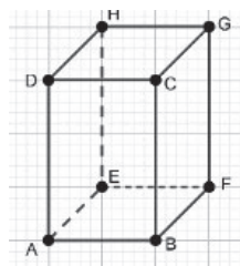
Paralelepípedo
