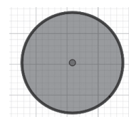
Círculo
