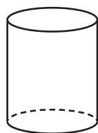
Cilindro
