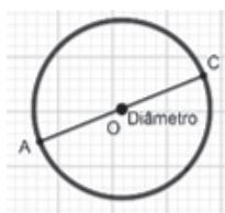
\overline{AC} - Diâmetro
