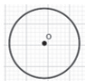
Circunferência
