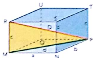
Paralelepípedo rectângulo de dimensões a , b e c , em que: D – diagonal do paralelepípedo; d – diagonal de uma face.
