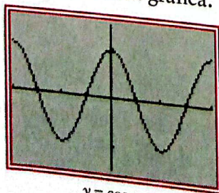
y = \cos x
