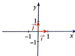
Referencial o. n. (O, \vec{i}, \vec{j})
