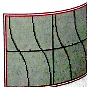
y = \cotan x
