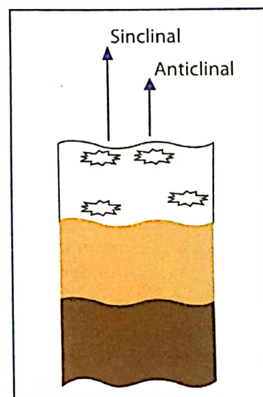
Fig. 134 Sinclinal/Anticlinal
