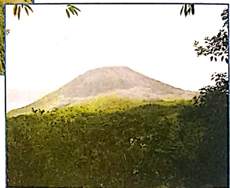
Fig. 140 Vulcão activo
