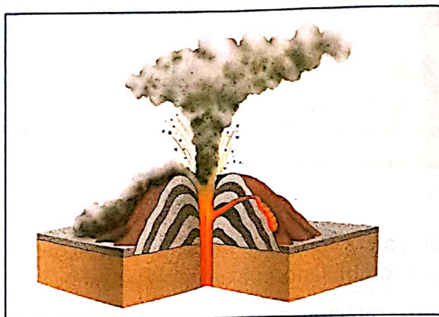
Fig. 145 Vulcão vulcaniano
